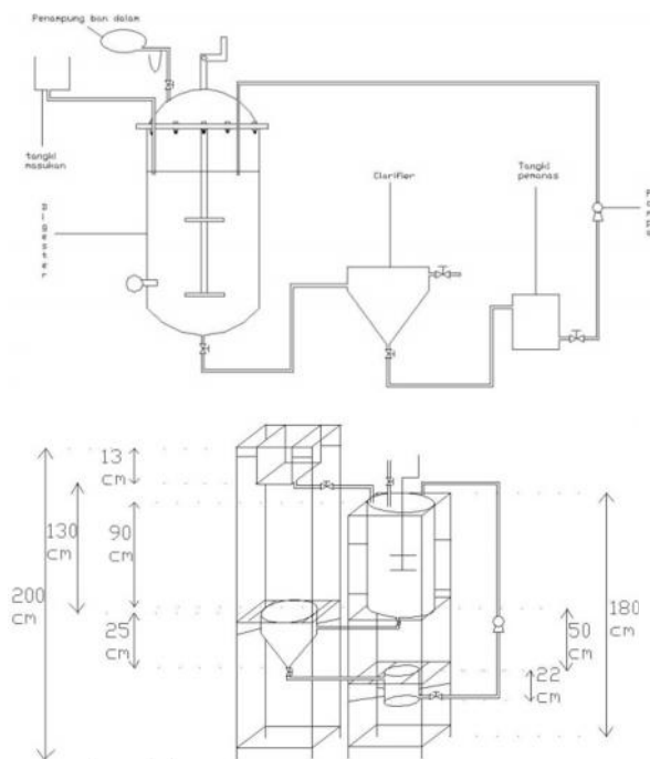
Gambar 1. Rangkaian Alat Proses
