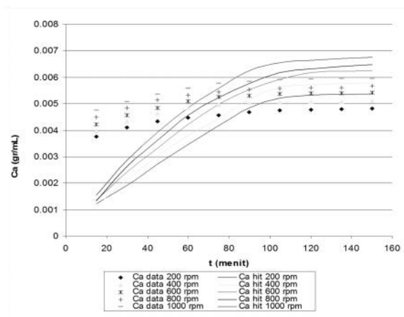
Gambar 1. Grafik hubungan antara Konsentrasi ( C_A ) dengan t (menit) pada Variasi Kecepatan Sirkulasi Pompa
