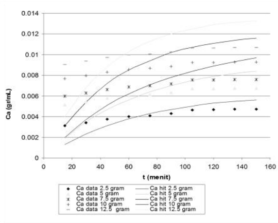
Gambar 2. Grafik hubungan antara Konsentrasi (Ca) dengan t (menit) pada Variasi Berat Pupuk Padat
