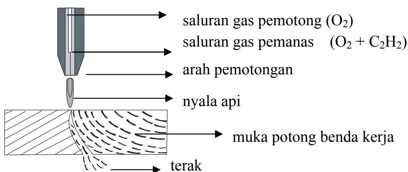
Gambar 4. Pemotongan dengan oksigen
