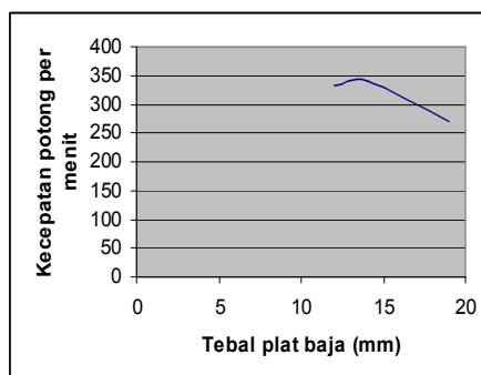
Gambar 13. Grafik kecepatan pemotongan plat baja
