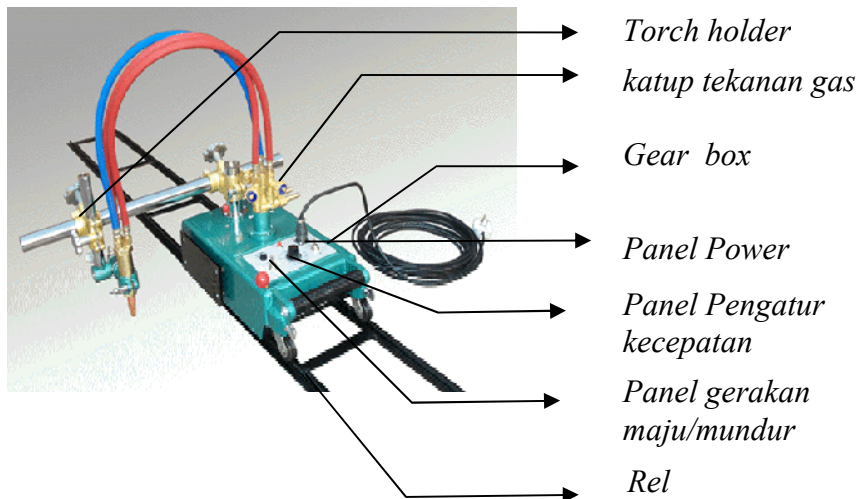
Gambar 10. Bagian-bagian dari Gas Cutting Machine
