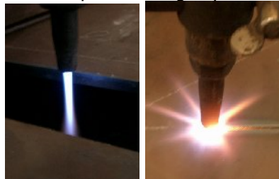
Gambar 7. Nyala api pemotongan
