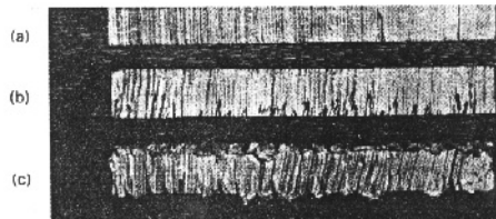
Gambar 5. Bentuk hasil pemotongan pada plat
