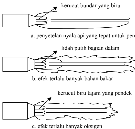
Gambar 6. Penyetelan nyala api
