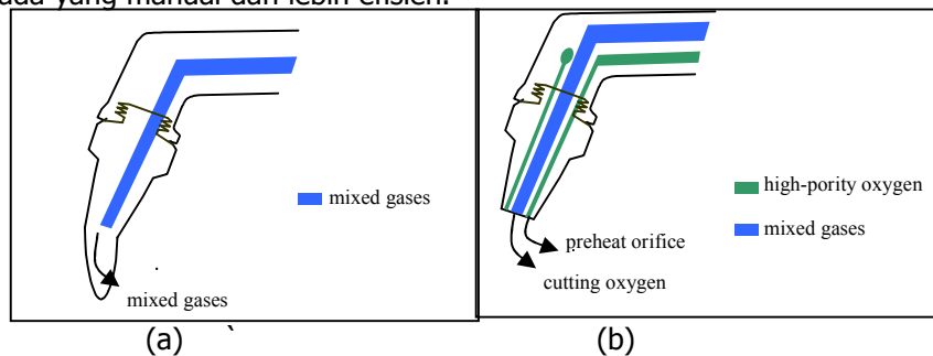
Gambar 3. Jenis Torch head (a) untuk pengelasan (b) untuk pemotongan
